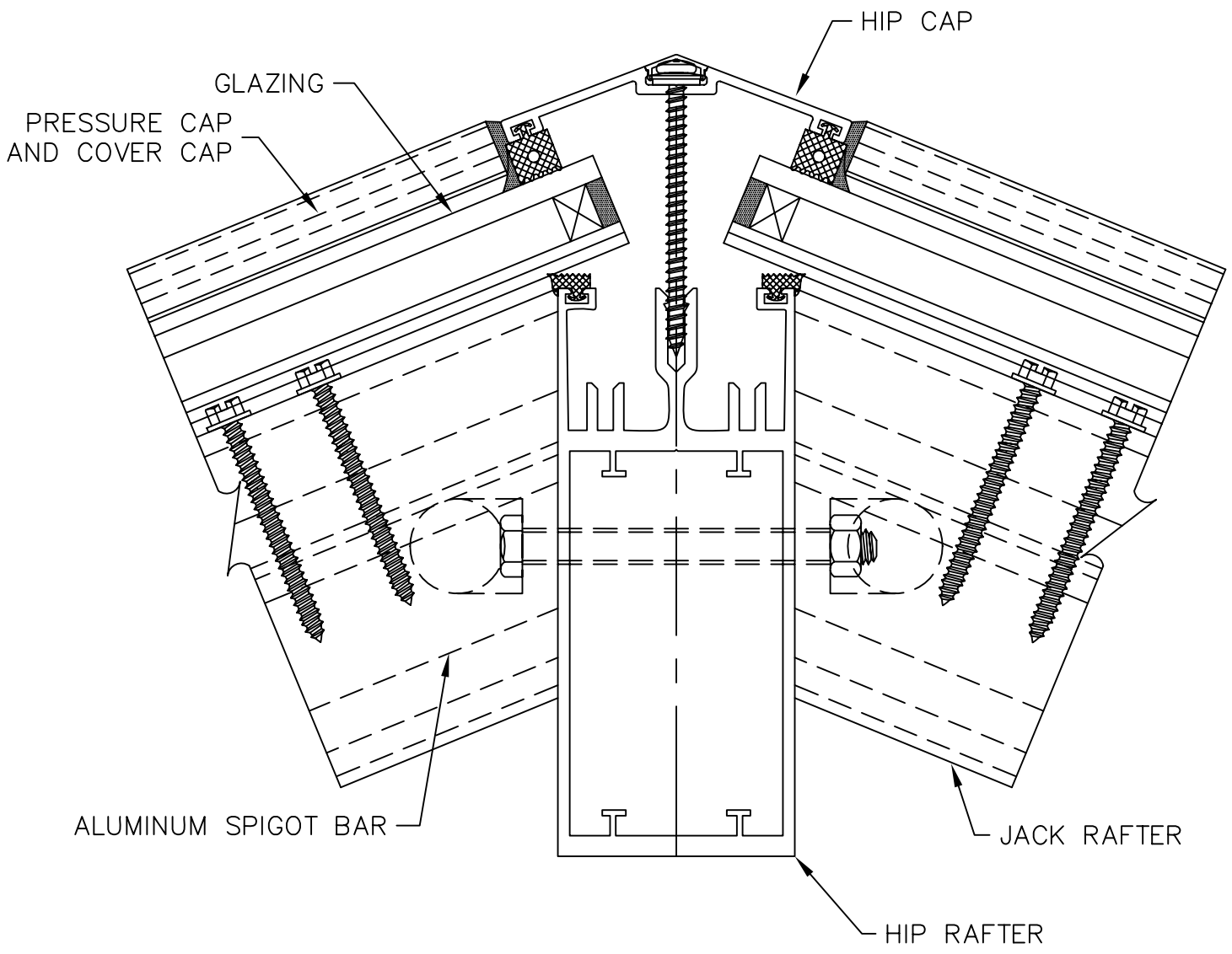
○ ———— HIP RAFTER ———— DETAIL
