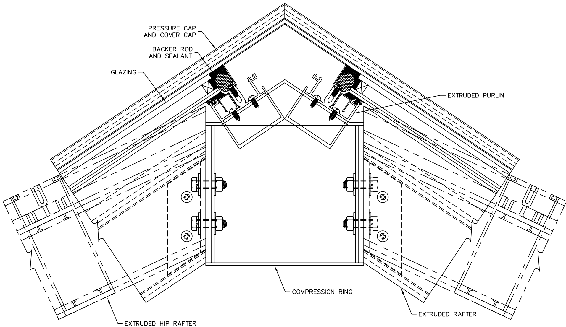
○ ——— RIDGE ———— DETAIL
